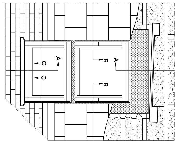
Eestvaade 1:20
